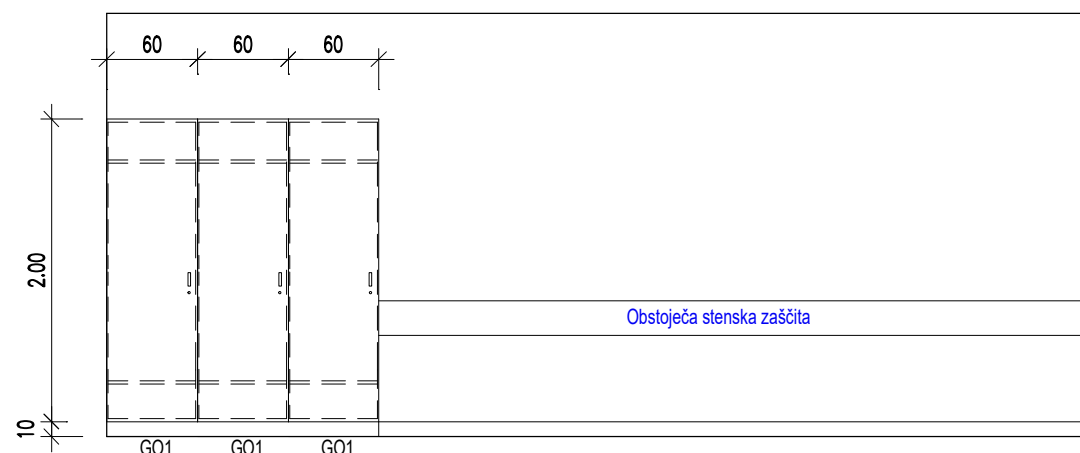
POGLED A
